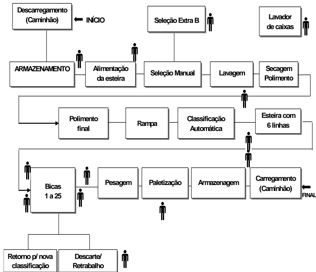
FIGURA 1 - Fluxo da produção em uma Unidade de Beneficiamento de tomates
